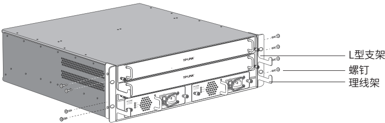
图2-1 理线架和L型支架安装示意图
